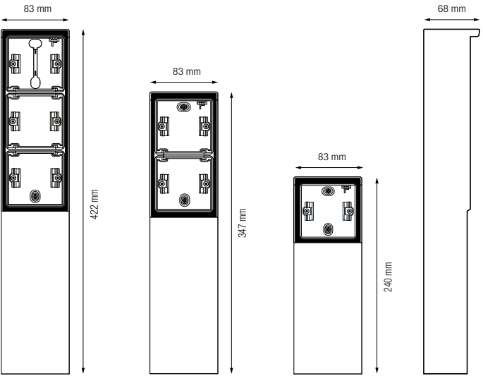
Baseplate
